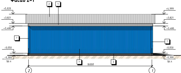
Фасад 2-1
