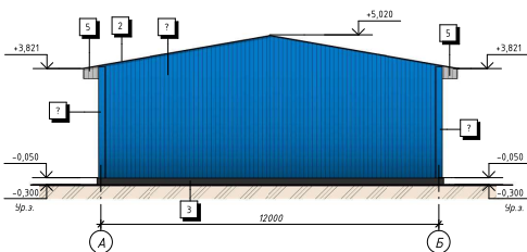
Фасад А-Б
