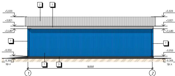
Фасад 1-2
