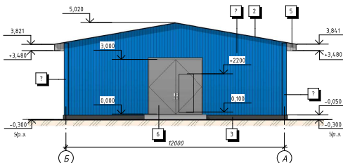
Фасад Б-А
